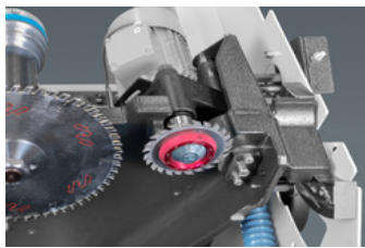
Voorritszaag Scoring saw Scie à inciser
