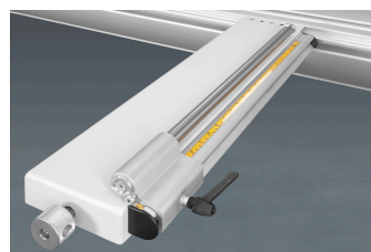
Extra steunafel met lengteaanslag Additional support table with length stop Table de support supplémentaire avec butée de longueur
