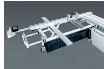
Z4 comfort afkorttafel 540 x 1440 mm met lengtecorrectie Z4 comfort cross-cut table 540 x 1440 mm with length correction Table à tronçonner confort Z4, 540 x 1440 mm avec correction de longueur
