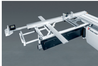
Z4 comfort afkorttafel 650 x 1415 mm met lengtecorrectie Z4 comfort cross-cut table 650 x 1415 mm with length correction Table à tronçonner confort Z4, 650 x 1415 mm avec correction de longueur
