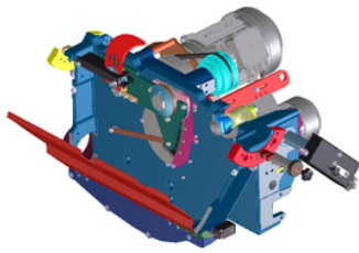
Stalen zaagaggregaat voor zaagblad dia 550 mm. Steel saw aggregate for saw blade dia 400 mm. Unité de scie en acier pour lame de scie de dia 400 mm.
