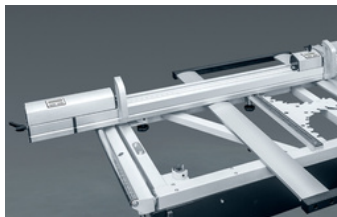
Digitale uitlezing op de flipper Z 5 (2 stuks) Digital readout on the flipper Z 5 (2 pieces) Affichage numérique sur butée Z 5 (2 pièces)
