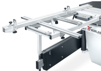
Z3 afkorttafel 540 x 970 mm, met telescopisch onder hoek uittrekbare korte (2050-3000 mm) Z4 aanslagbalk voorzien van twee aanslagen. Z3 cross-cut saw table 540 x 970 mm, with short (2050-3000 mm) Z4 telescopic, inclined fence, equipped with two stops. Table à tronçonner Z3, 540 x 970 mm, avec court (2050-3000 mm) Z4 guide télescopique inclinable, équipée de deux butées.
