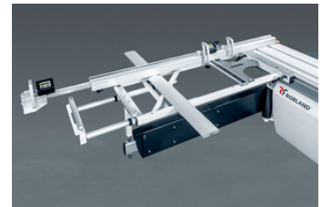
Z4 comfort afkorttafel 540 x 1440 mm met lengtecorrectie Z4 comfort cross-cut table 540 x 1440 mm with length correction Table à tronçonner confort Z4, 540 x 1440 mm avec correction de longueur
