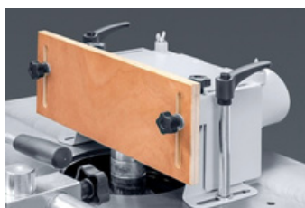
Pennenkap voor snijgereedschappen tot dia 250 mm Tenoning safety hood for cutting tools up to dia 250 mm Capot à tenonner (diam. outil 250 mm)
