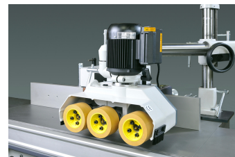
Aandrijver met 3 wielen: RAV32 of RAV33 Feeder with 3 wheels: RAV32 or RAV33 Entraîneur avec 3 rouleaux: RAV32 ou RAV33
