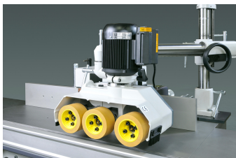
Aandrijver met 3 wielen: RAV32 of RAV33 Feeder with 3 wheels: RAV32 or RAV33 Entraîneur ave 3 rouleaux: RAV32 ou RAV33
