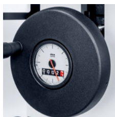
Handwiel met uitleesklok schaaft hoogte Handwheel with readout planing height Volant avec vernier, réglage en hauteur raboteuse
