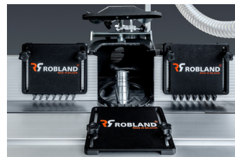
Featherboard voor loopwagen of freeskap Featherboard for standard fence or sliding table Planches à plumes pour chariot ou toupie
