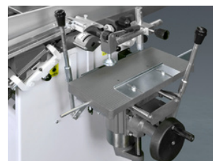
Langgatboor incl. houtklem Mortising unit, wood clamp included Mortaiseuse avec presseur à bois inclus
