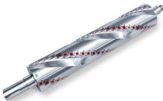
Spiraal schaafas 410 x 70 mm, 68 messen Spiral planing shaft 410 x 70 mm, 68 knives Arbre de rabotage hélicoïdal 410 x 70 mm, 68 plaquettes
